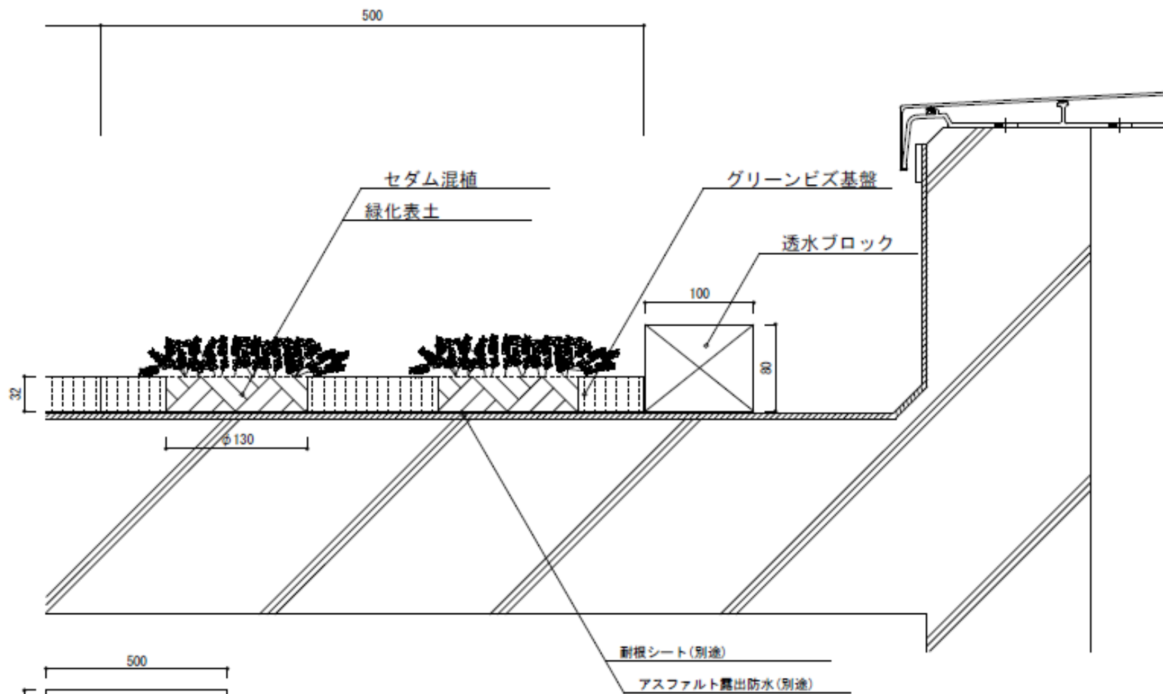
断面図 A4 : 1 / 5
