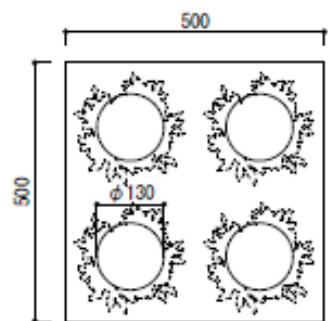
平面図 A4 : 1 / 15
